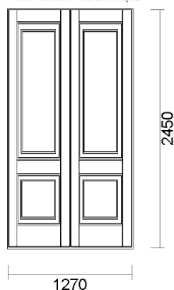
Widok stolarki od zewnątrz
